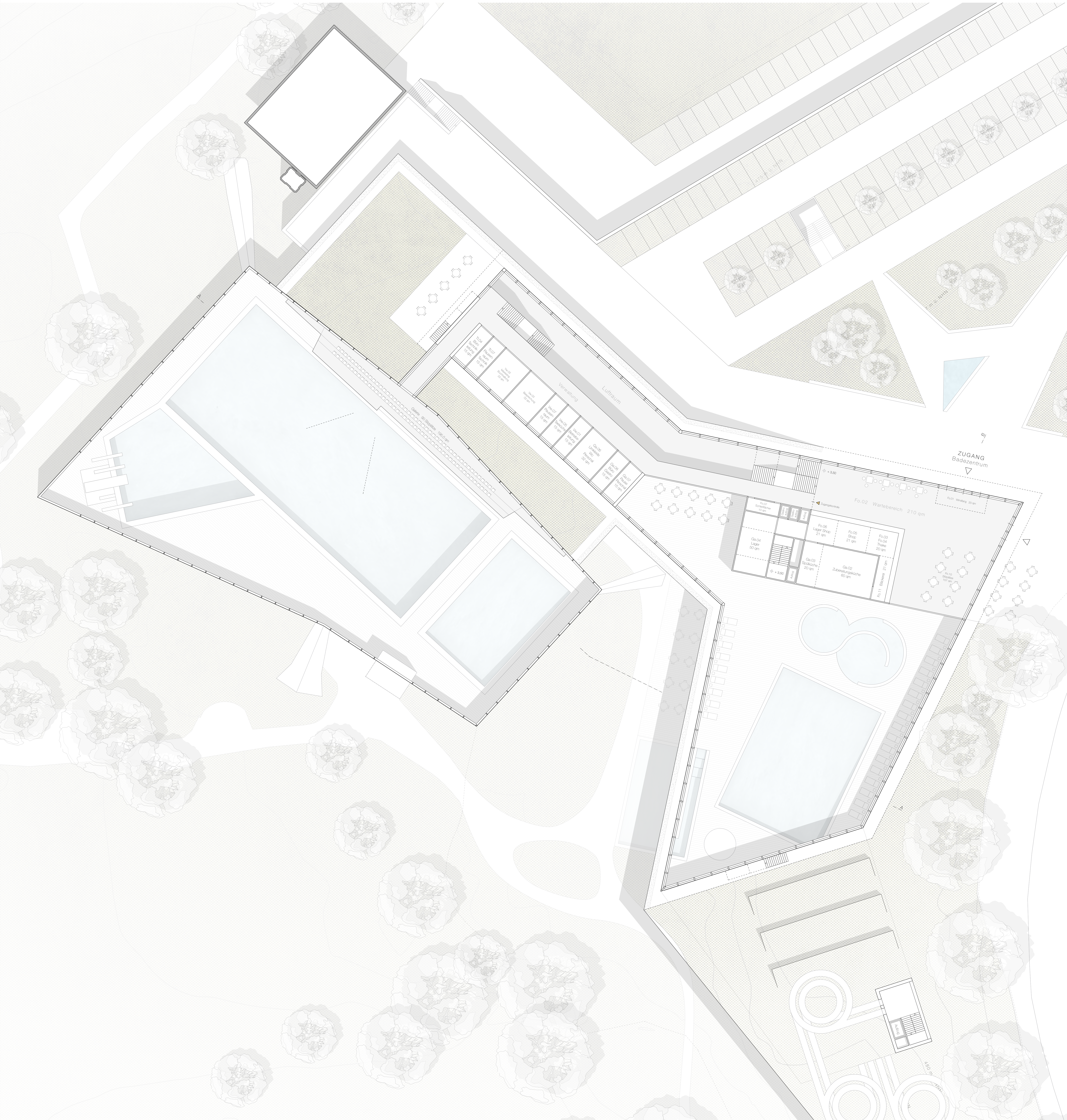
Grundriss Erdgeschoss 1:200
