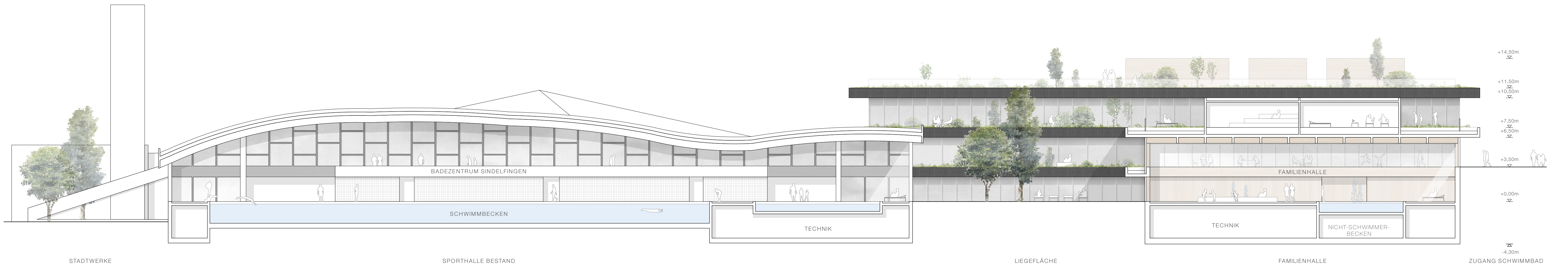
Schnitt A-A 1:200
