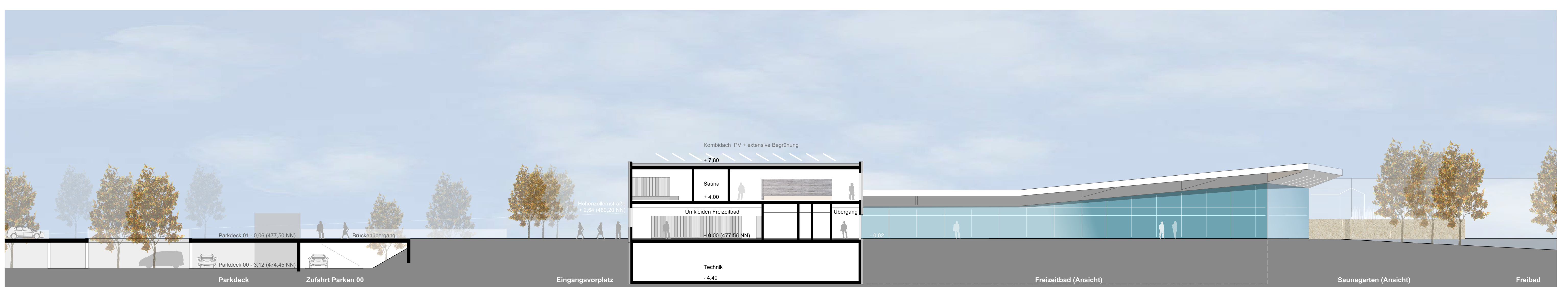
Schnitt Umkleebereich Familienbad M 1 200
